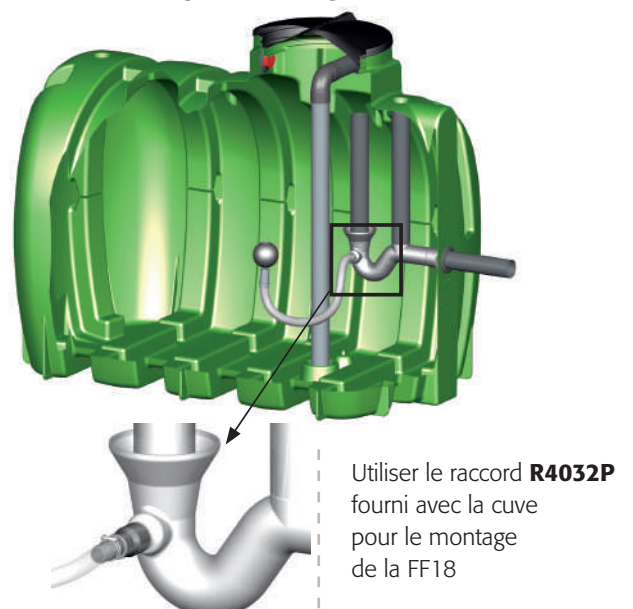
Montage version stockage et rétention
