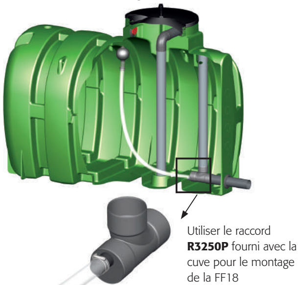
Montage version rétention
